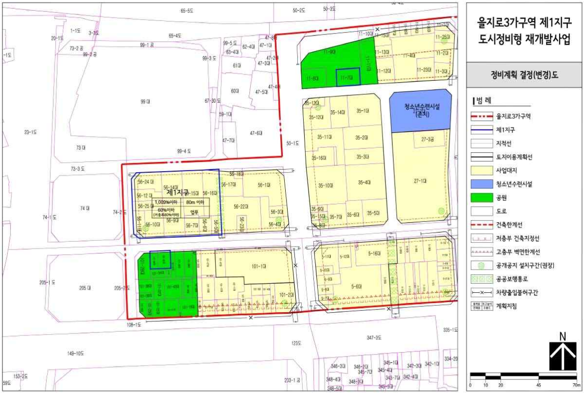
<정비계획 결정(변경)도>
