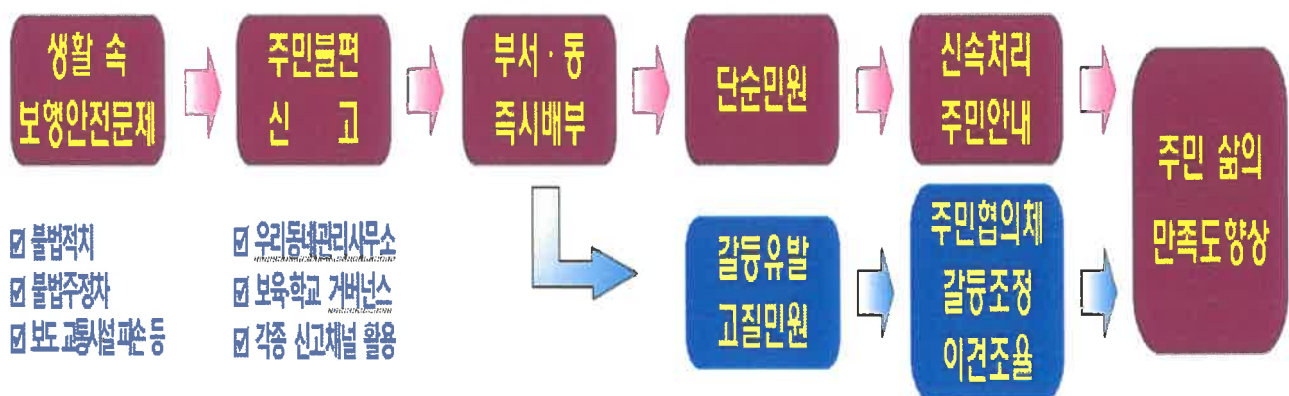
〈거버넌스 운영체계도〉
